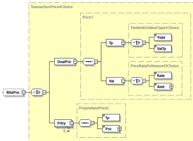
Abbildung 116: camt.053.001.08, RltdPric
