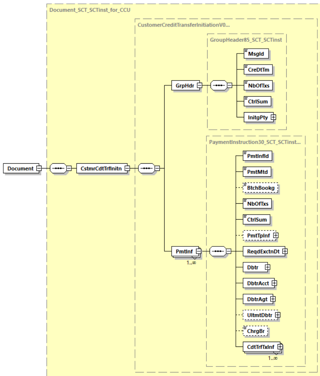
Abbildung 138: Übersicht pain.001.001.09
