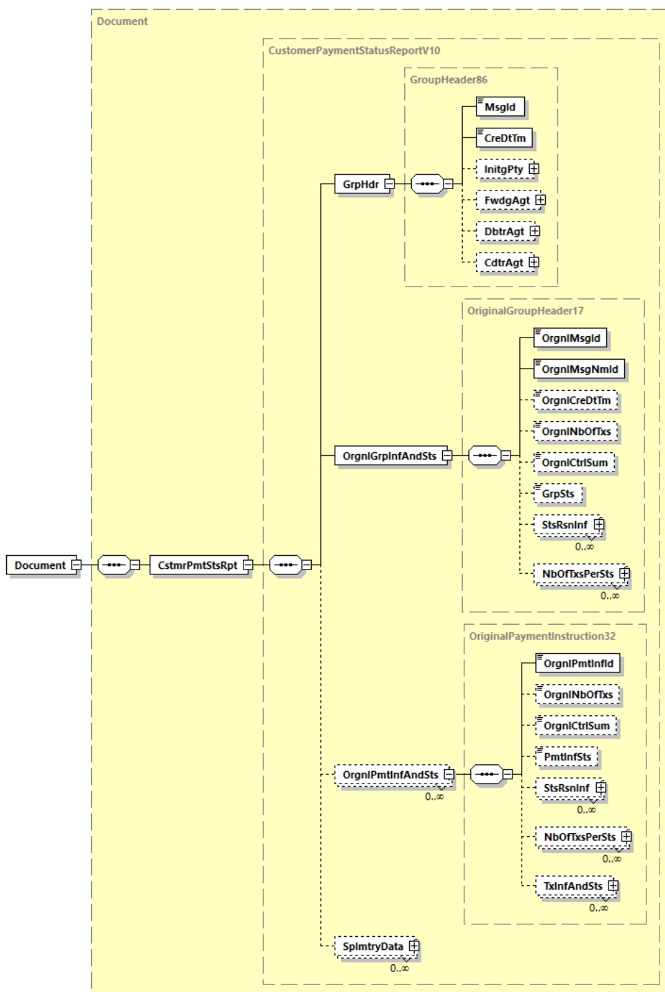
Abbildung 64: Übersicht pain.002.001.10
