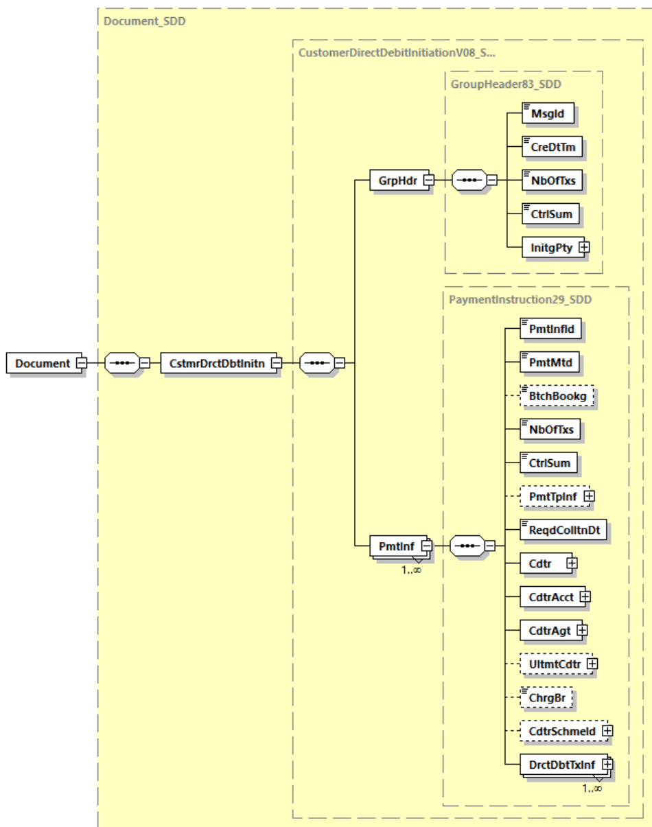
Abbildung 31: Übersicht pain.008.001.08
