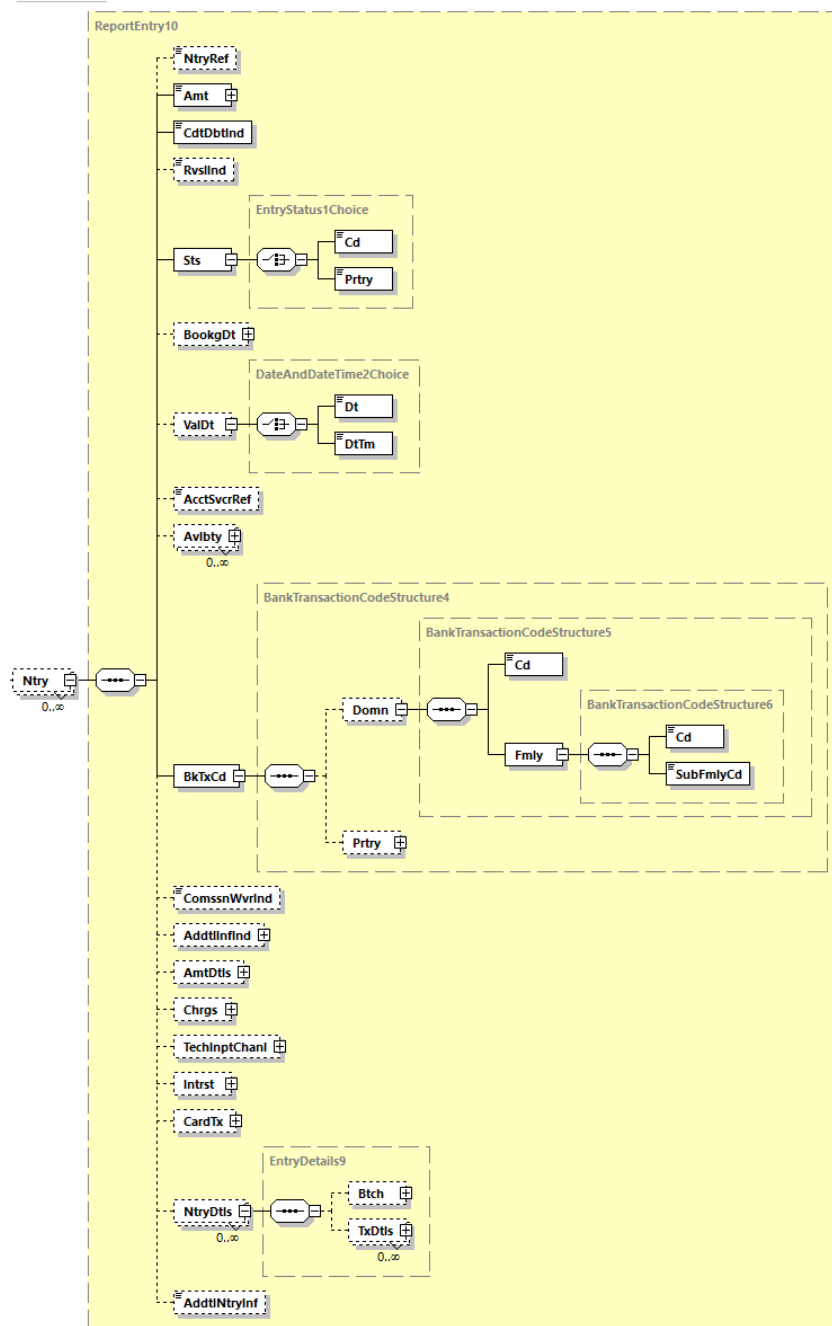
Abbildung 60: camt.054.001.08, Ntry
