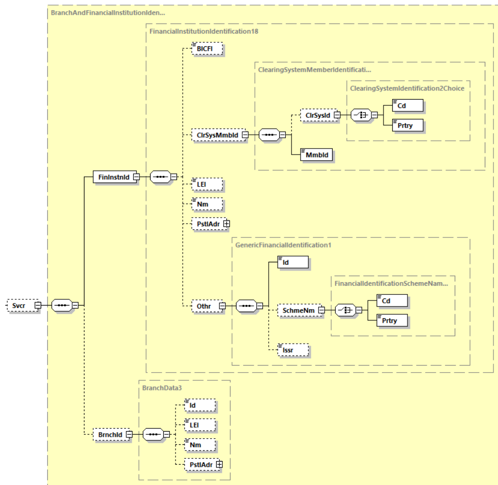
Abbildung 106: camt.053.001.08, Svcr
