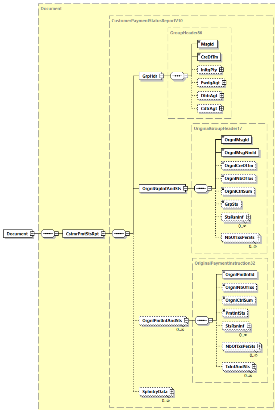
Abbildung 43: Übersicht pain.002.001.10
