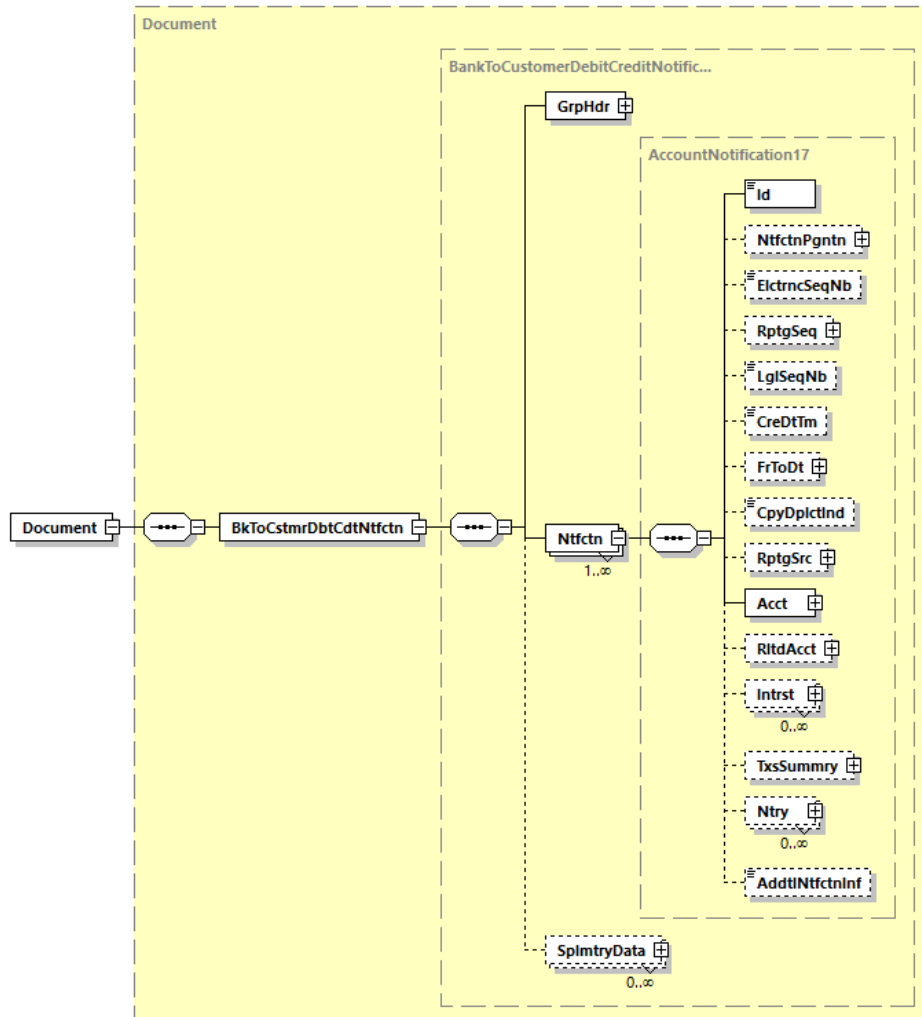
Abbildung 133: Übersicht camt.054.001.08
