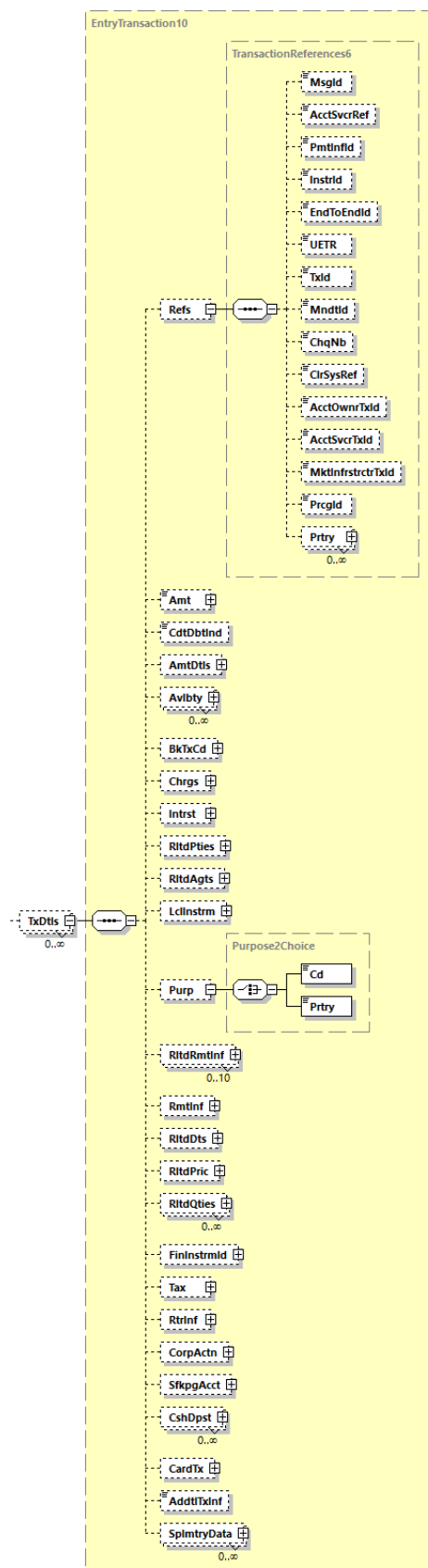
Abbildung 61: camt.054.001.08, TxDtls
