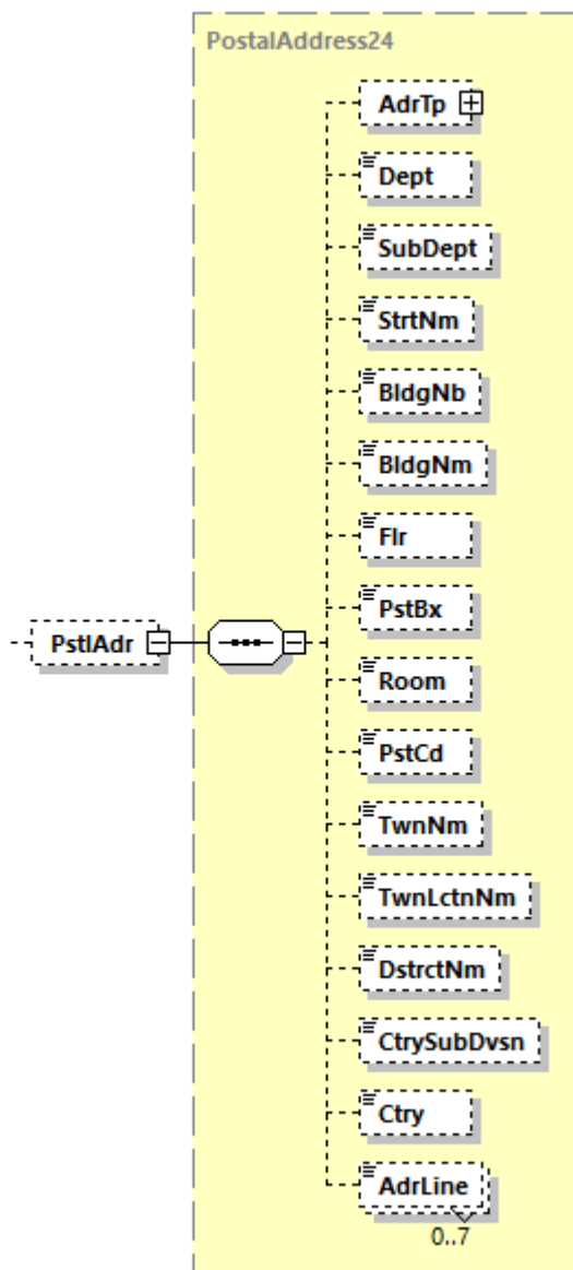
Abbildung 123: camt.053.001.08, PstlAdr
