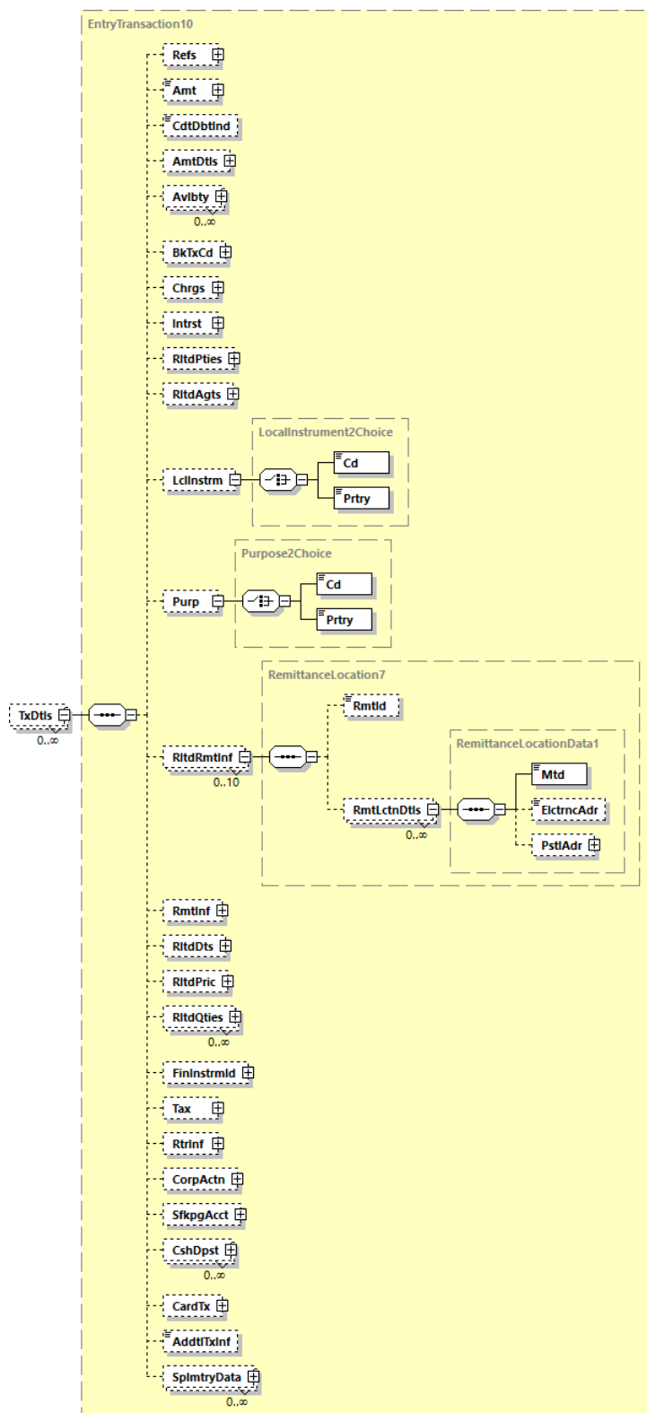
Abbildung 108: camt.053.001.08, TxDtIs
