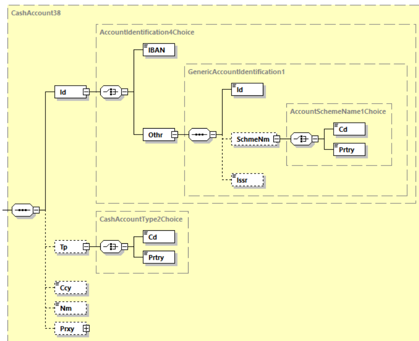
Abbildung 126: camt.053.001.08, CashAccount38
